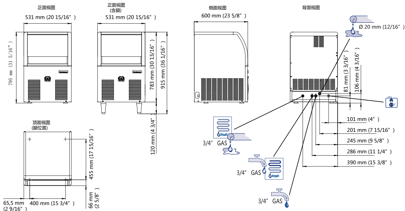
AC 86 风冷
