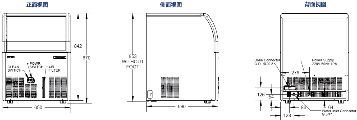
装矮腿式样
